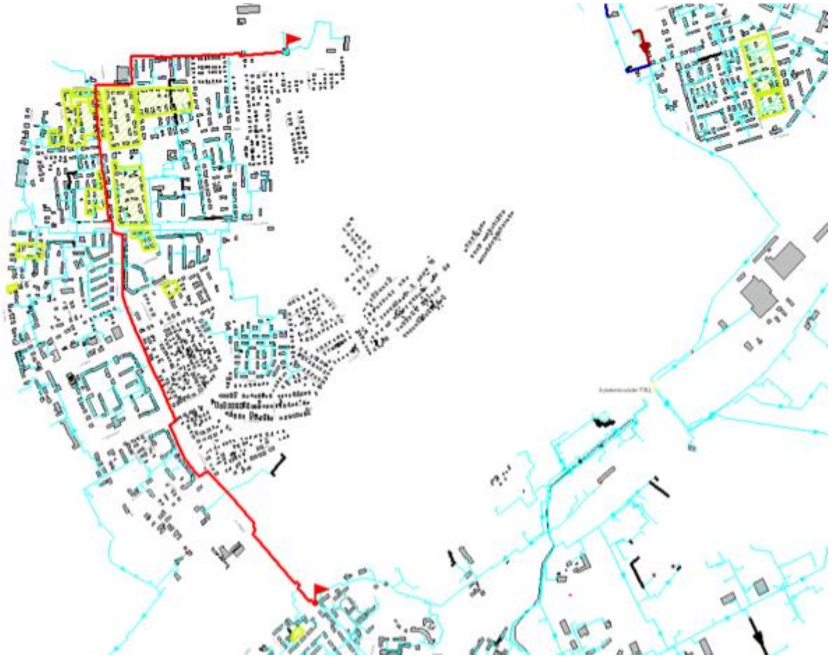
Рисунок 3.1 – Путь для расчёта вероятности безотказной работы тепловых сетей от ТК-45 до С-28п-16
